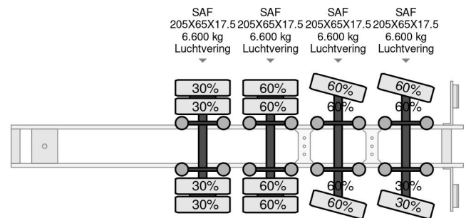
Nootboom OSD-50-04V 2 AXLE STEERING. 6,7 METER E...
